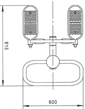
Рисунок 2 - Вид сверху
